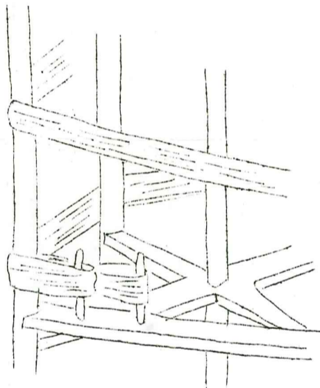
Fig 20. Varpa: detalj (Dal.) (skälträ o. skälpinningar)
